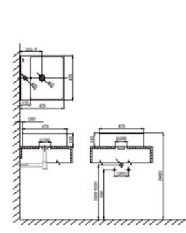
47cm Vessel Basin (1-Hole) Size: 470x470x170mm Material: Vitreous china 47公分台上盆 (单孔) 尺寸: 470x470x170mm 材质: 陶瓷
