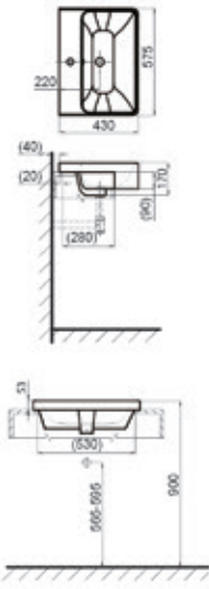
58cm Semi-Recessed Basin (1-Hole) Size: 575x430x170mm Material: Vitreous china 58公分半嵌盆(单孔) 尺寸: 575x430x170mm 材质: 陶瓷
